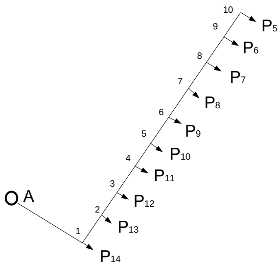
Рисунок 6 Розрахункова схема лінії (фідера) живлення споживачів
