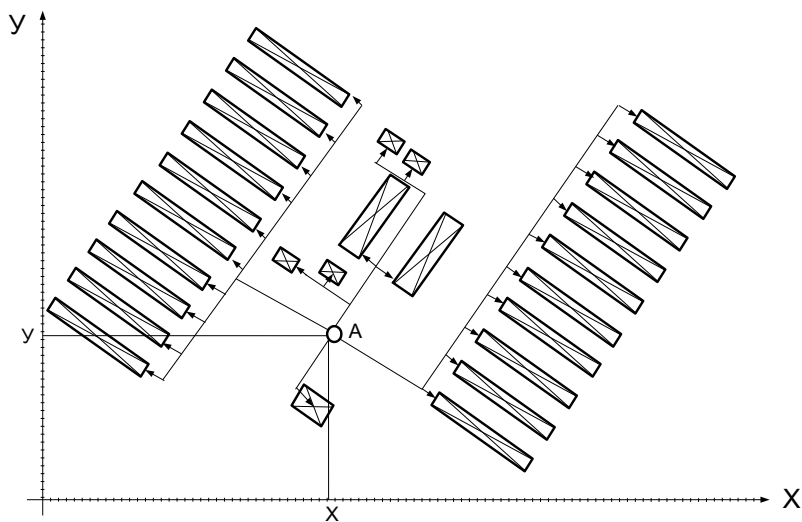
Рисунок 4 План господарства із нанесенням ЛЕП 0,4кВ від трансформаторної підстанції А
