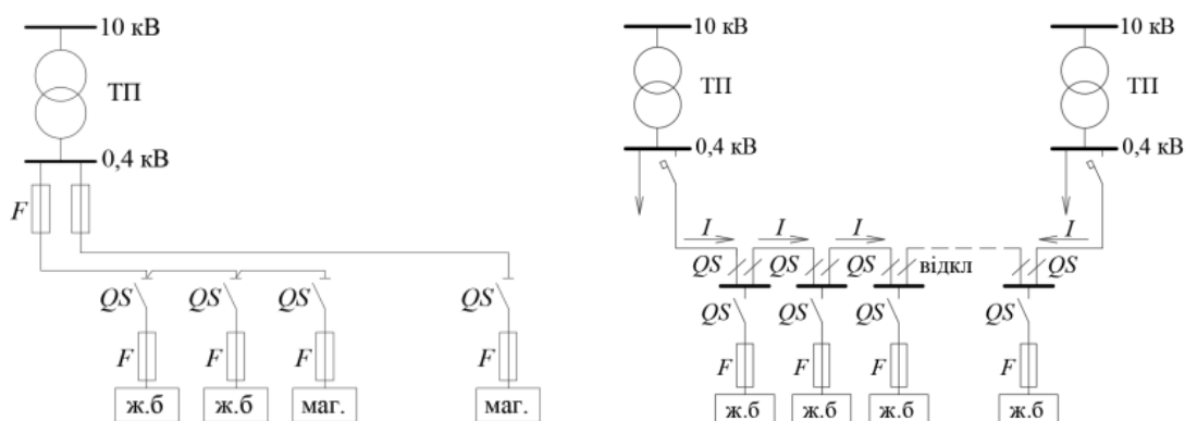
Рисунок 1 Радіальна та петльова схеми низьковольтної мережі
