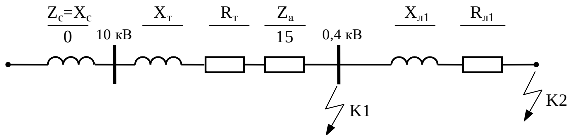
Рисунок 8 Еквівалентна схема заміщення Фідера 1
