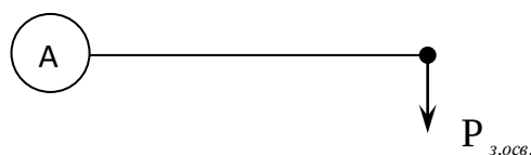
Рисунок 7 Розрахункова схема зовнішнього освітлення фідерів
