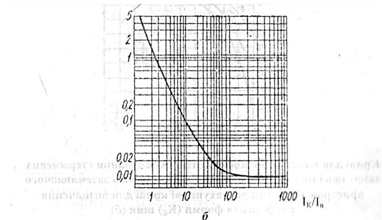
Ампер-секундна характеристика запобіжників ПК 10 (а), характеристика найбільшого часу горіння дуги ( t_{ад} ) запобіжників ПК 10 (б)
